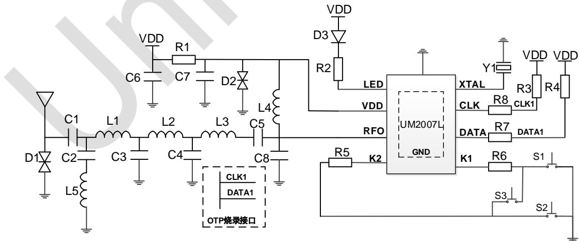
图 7-2：按键扫描模式应用原理图
