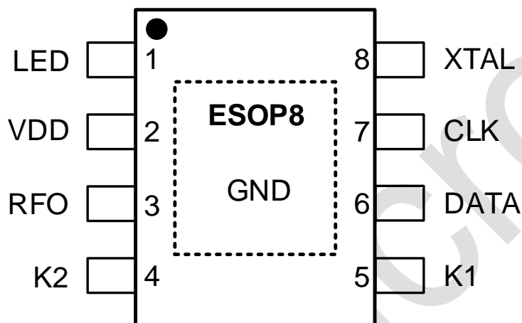
图 3-1：ESOP8 封装管脚分布图
