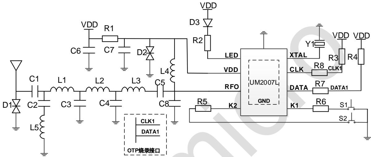
图 7-1：普通按键模式应用原理图
